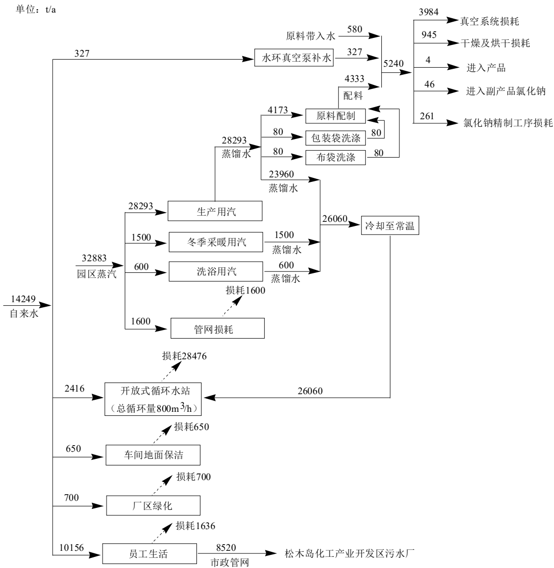
图2-7 全厂水平衡（现有工程+在建工程）图
